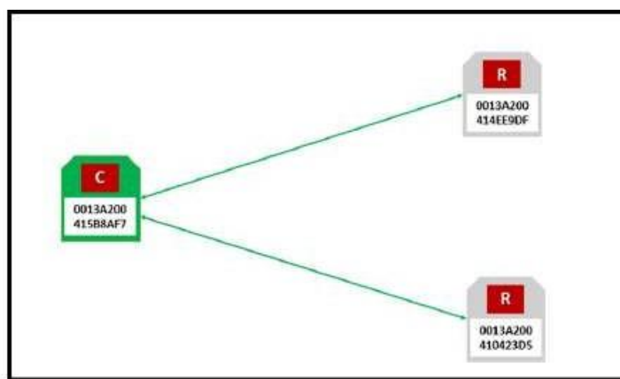
Gráfico 10. Topología de la red Fuente: Elaboración propia
